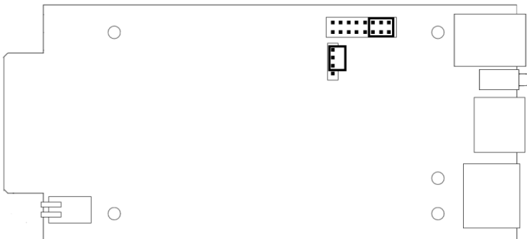
Abbildung 148: CS121 WDP PIN-Verbindung, Draufsicht
