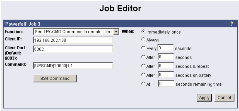
Abbildung 67: HTTP - Job Editor: RCCMD-Befehl
