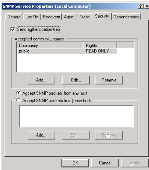
Abbildung 152: SNMP Dienst Eigenschaften
