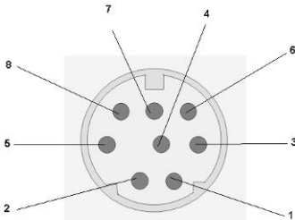
Abbildung 140: Pin COM2 Mini-DIN 8 pol
