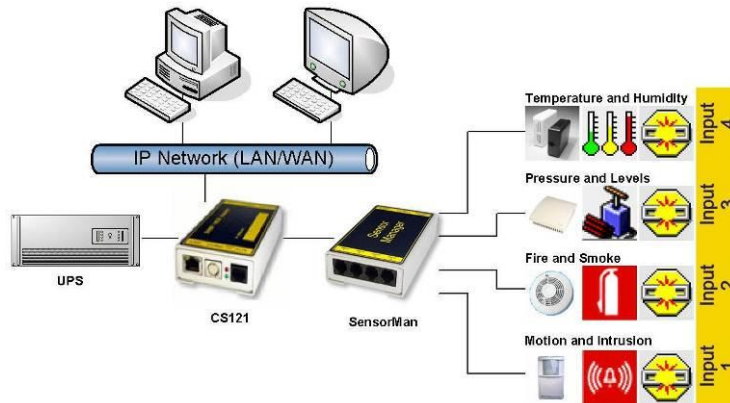
Abbildung 104: CS121-Installation mit SENSORMANAGER
