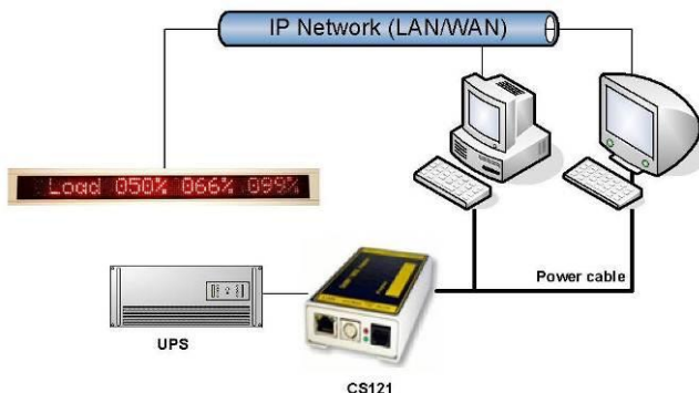
Abbildung 120: LED-Matrix Anzeige – Netzwerkintegration
