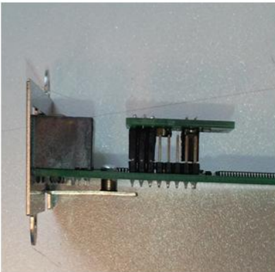
Abbildung 147: CS121 WDP auf einem CS121 SC/BSC – Ansicht von links und von hinten
