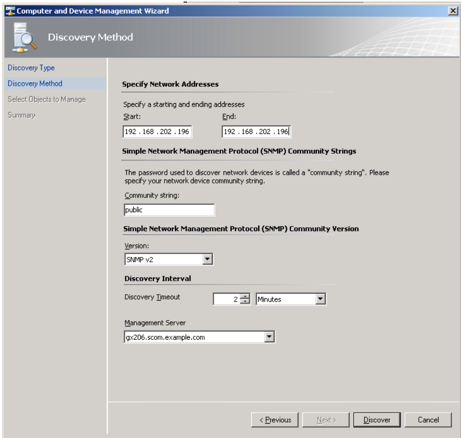
Abbildung 162: Discovery Method Fenster
