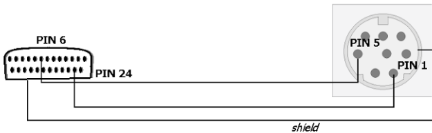
Abbildung 151: MODBUS - Cable 112
